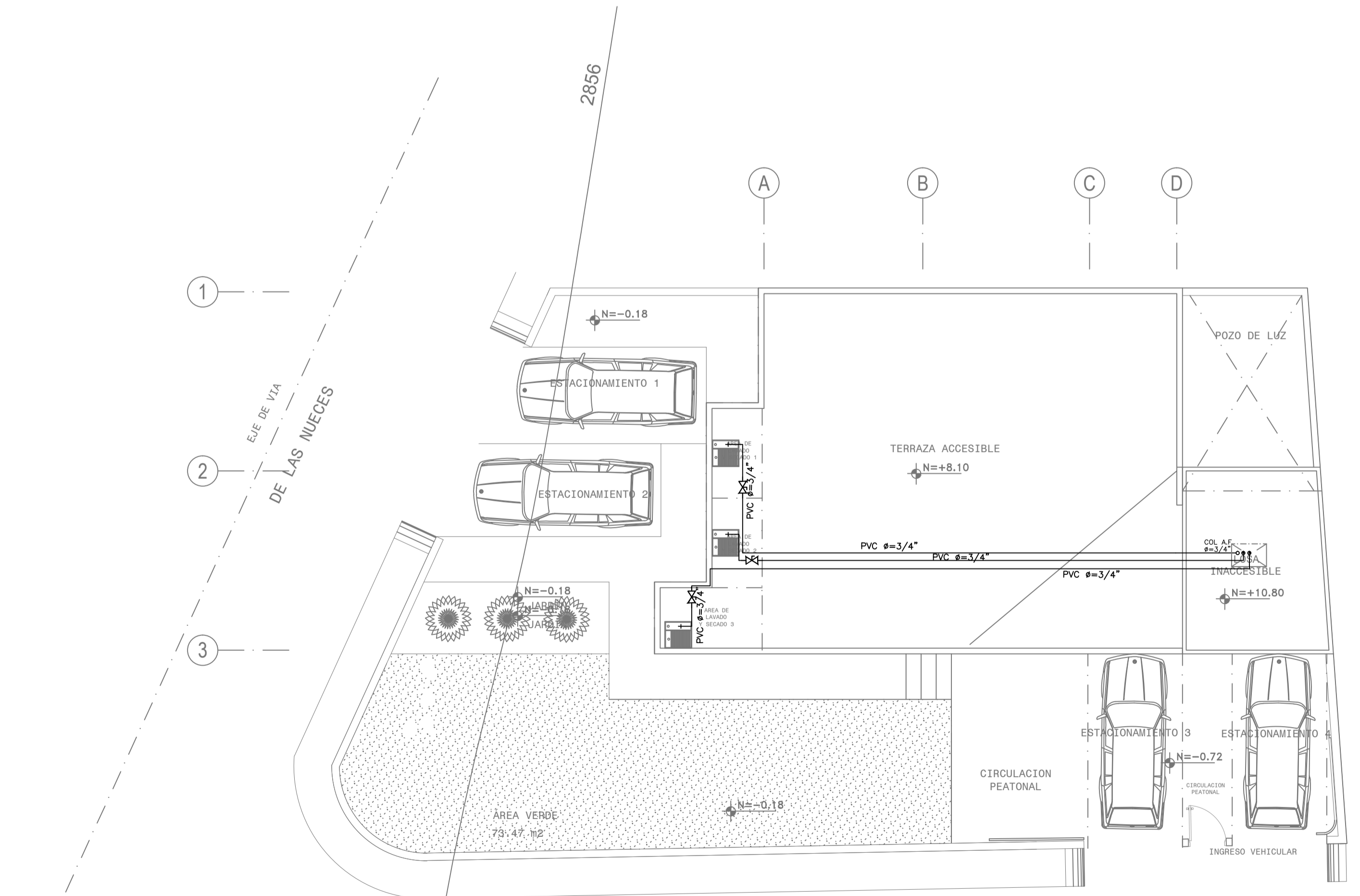
PLANTA DE CUBIERTA ESCALA-----1:100
