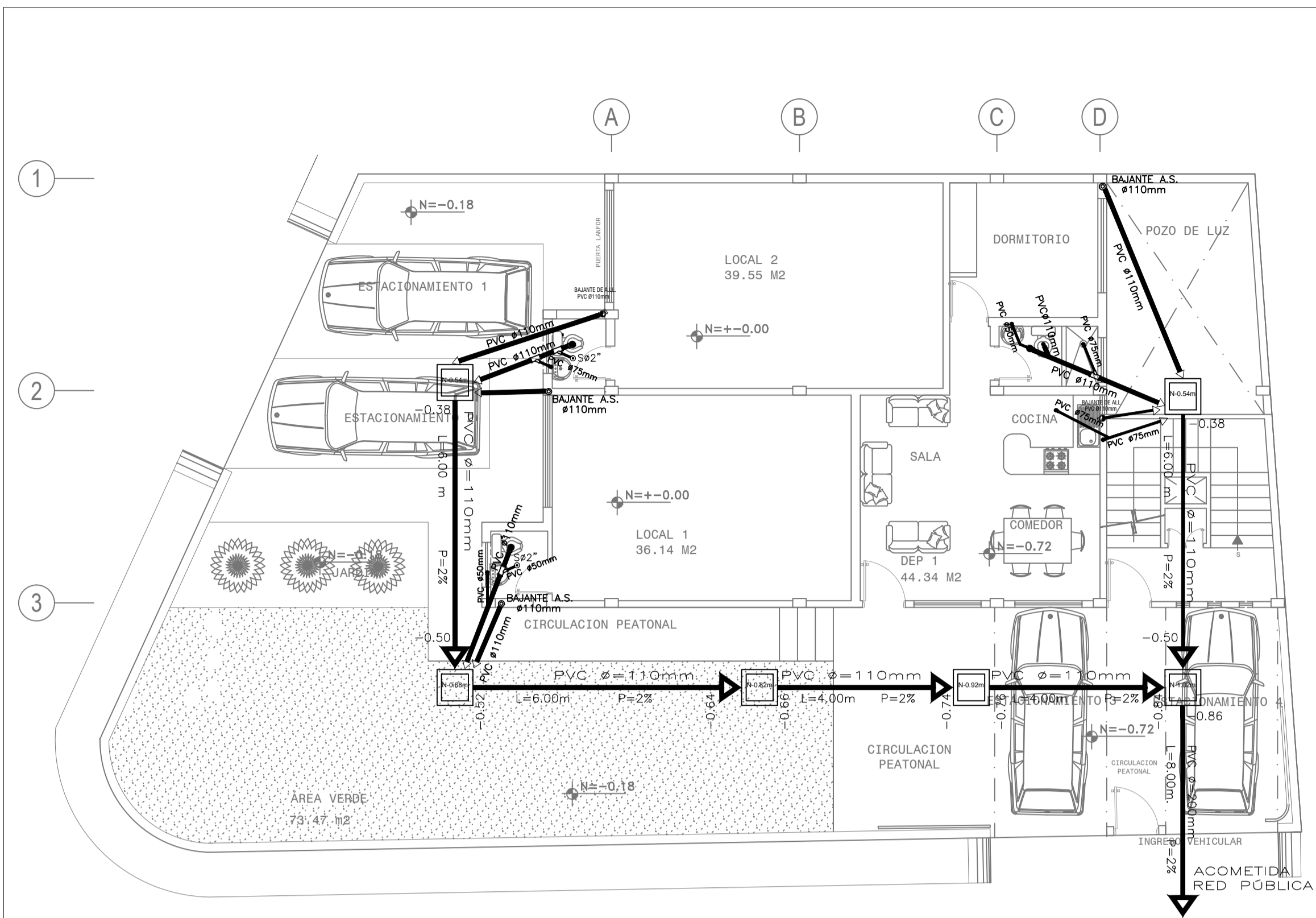
PLANTA BAJA ESCALA-----1:100
