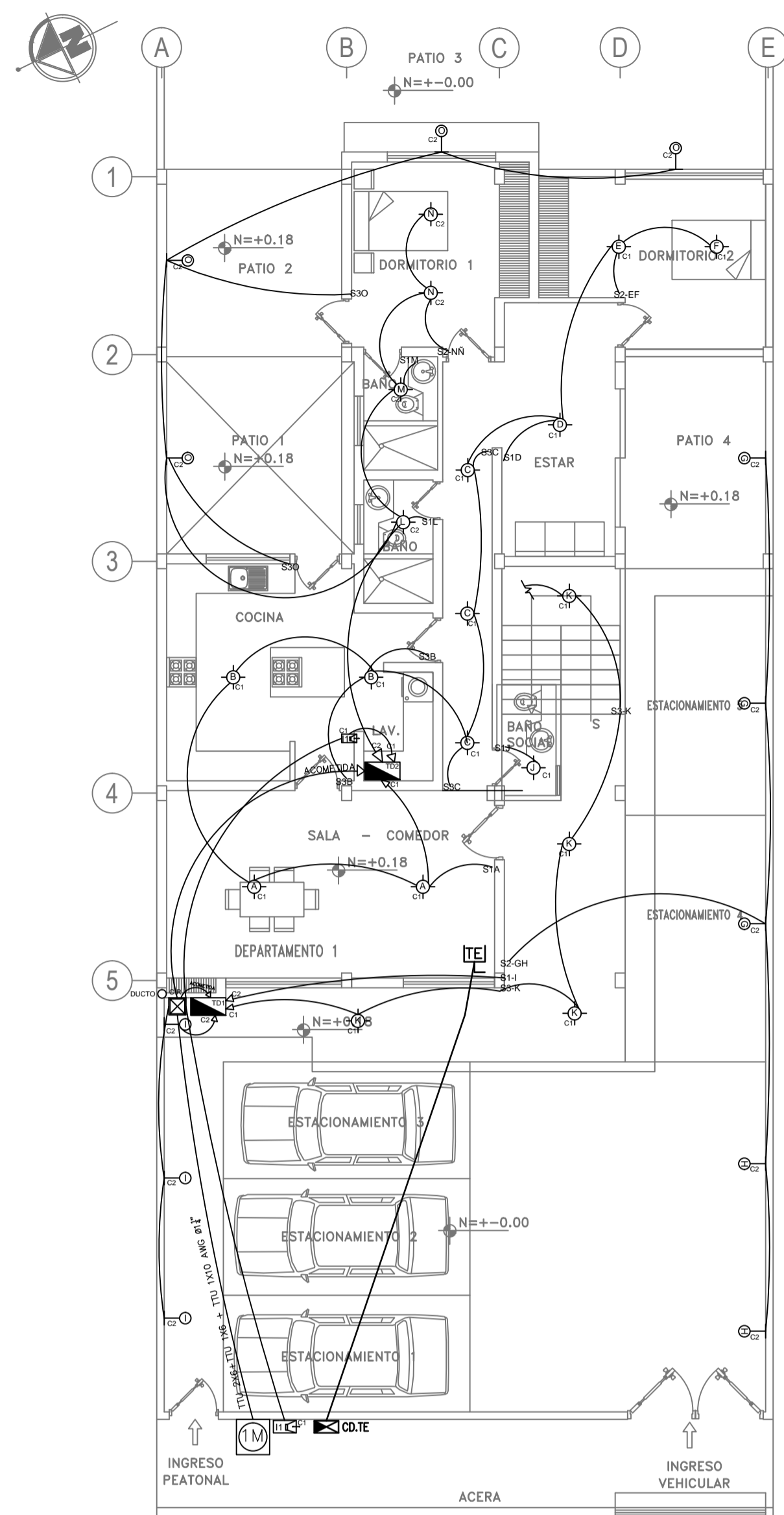
PLANTA BAJA INSTALACIONES ELÉCTRICAS ESCALA-----1:100
