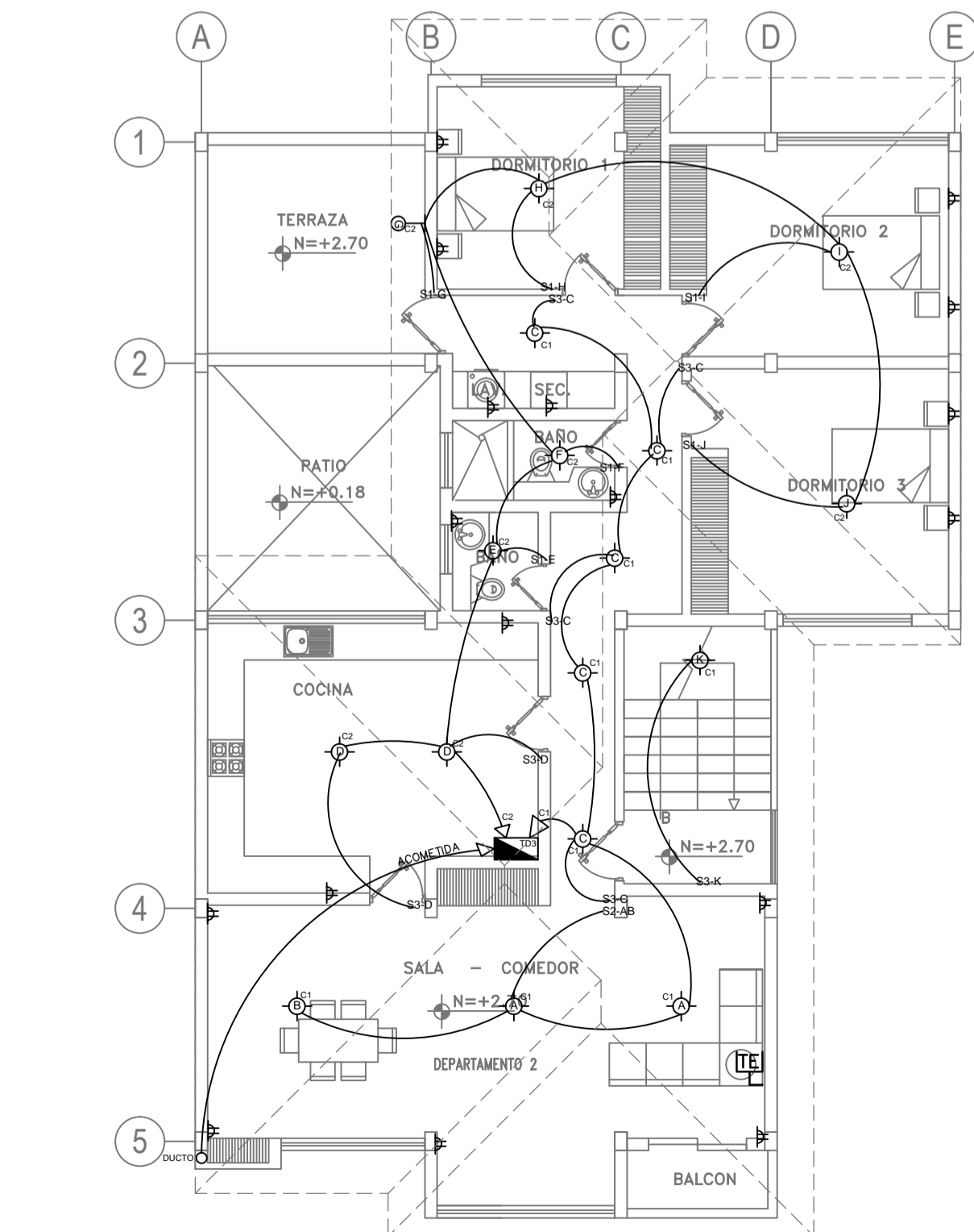
SEGUNDA PLANTA ALTA INSTALACIONES ELÉCTRICAS ESCALA-----1:100
