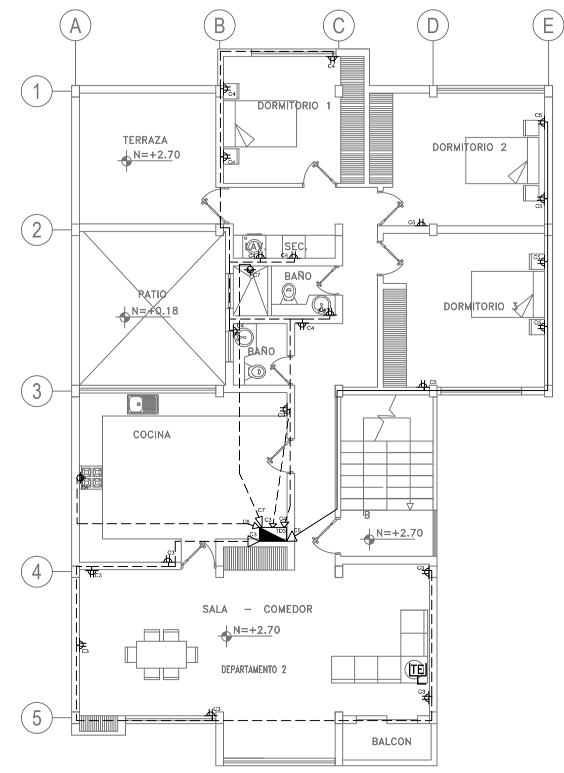
PRIMERA PLANTA ALTA INSTALACIONES ELÉCTRICAS ESCALA-----1:100
